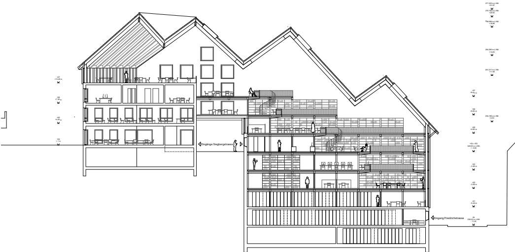
Schnitt Kölner Strasse - Friedrichstrasse M 1:200
