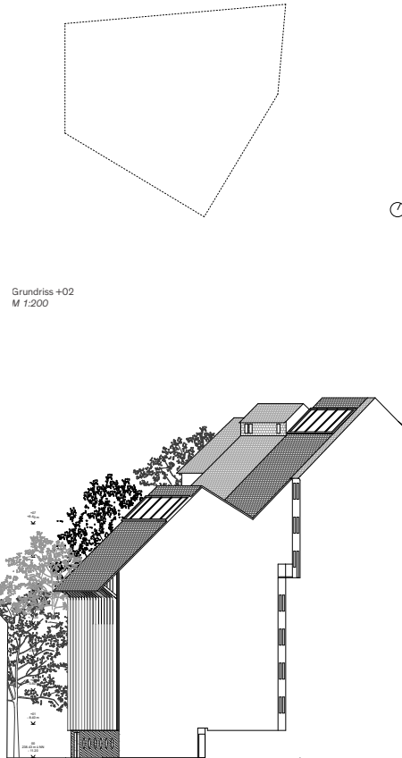
Ansicht Kölner Strasse M 1:200
